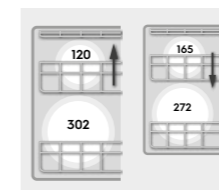
Maximale Tellergrössen EURO-Norm-Geschirrspüler mit 14 Massgedecken und ComfortLift*
